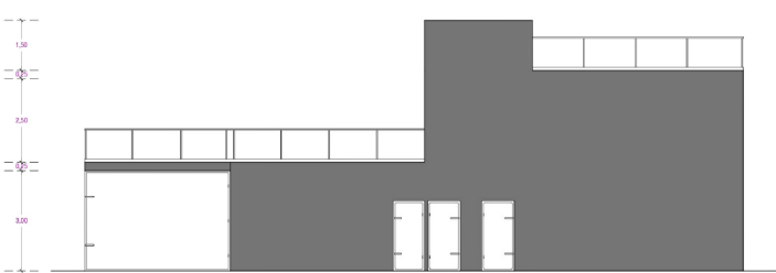
ESPAZO TERRA - PRÁCTICAS - FACHADA LATERAL DEREITA E.: 1/ 250
