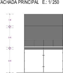
ESPAZO TERRA - PRÁCTICAS FACHADA PRINCIPAL E.: 1/ 250
