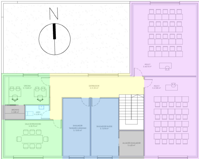
ESPAZO TERRA - AULAS - PLANTA PRIMEIRA E.: 1/ 200
