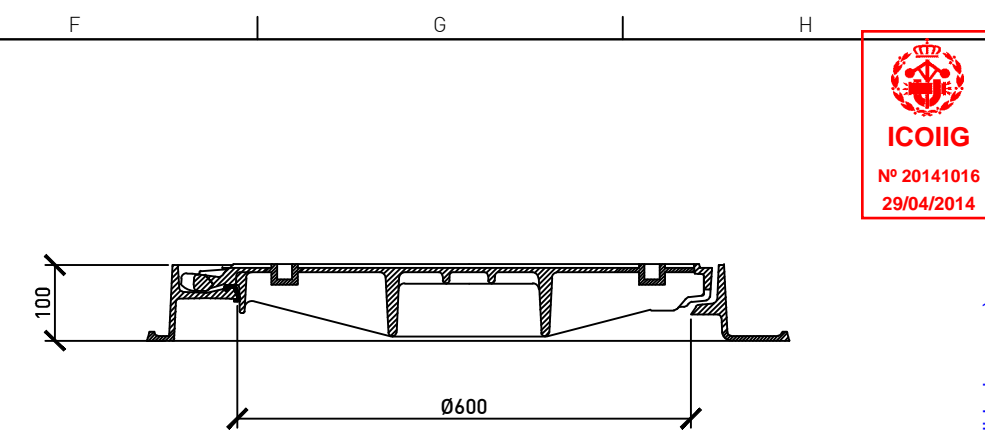
Sección A-A'
