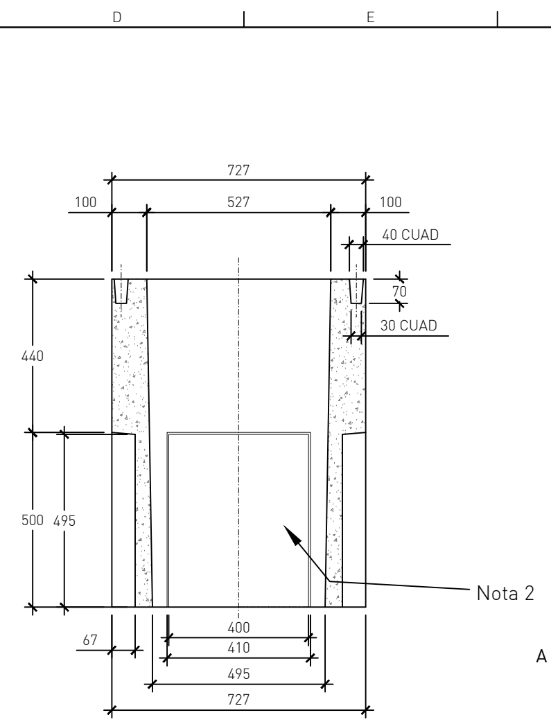
SECCION B-B
